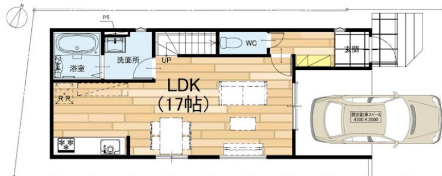
1階 平面図
