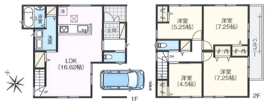
【間取り図】
