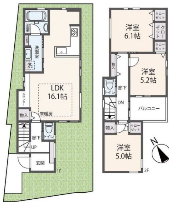
【間取り図】
