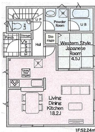
【間取り図】
