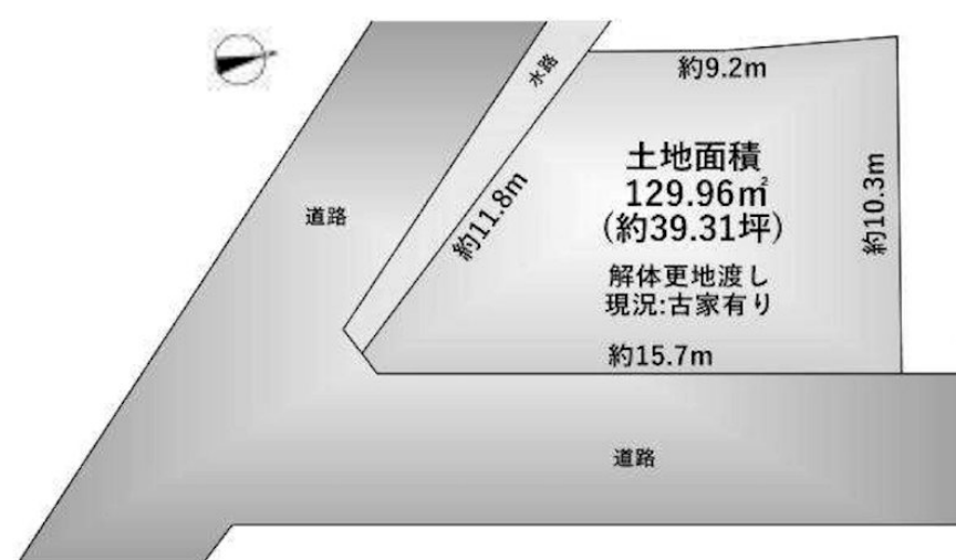
【区画図】
