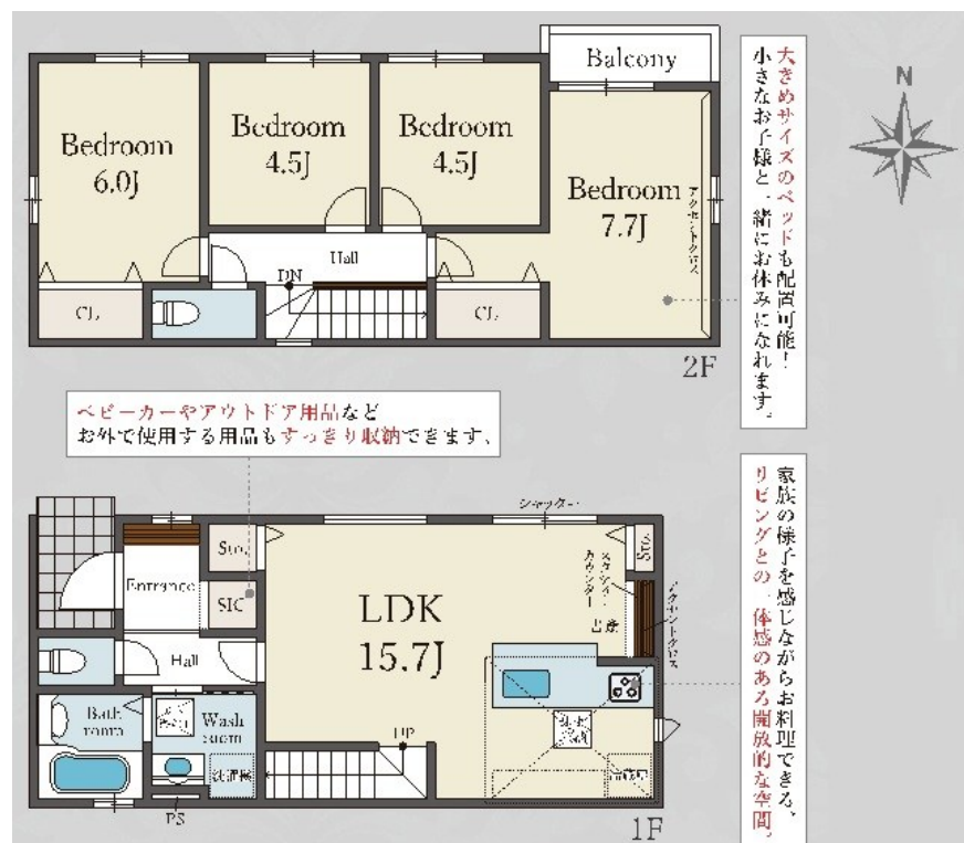
【間取り図】
