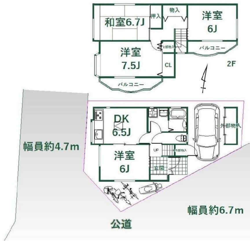
【間取り図】
