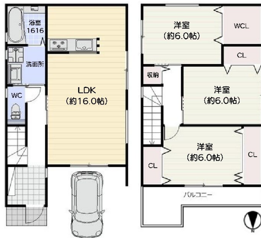
【間取り図】
