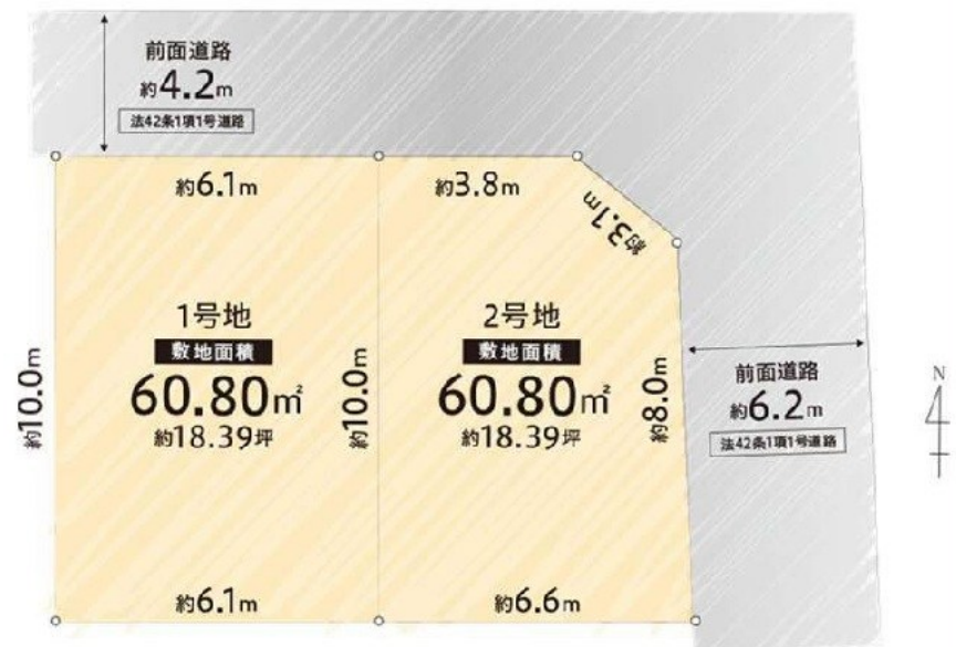
【区画図】
