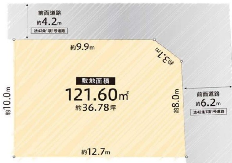
【区画図】
