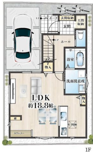
【間取り図】
