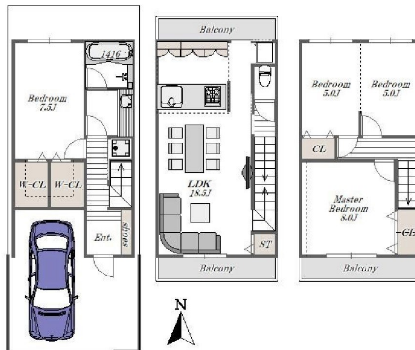
【間取り図】
