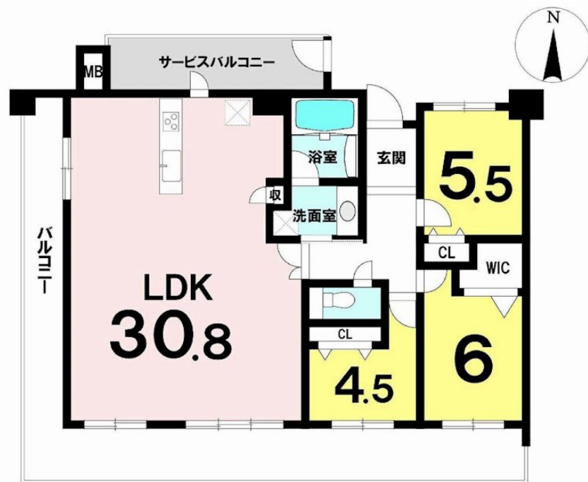
【間取り図】
