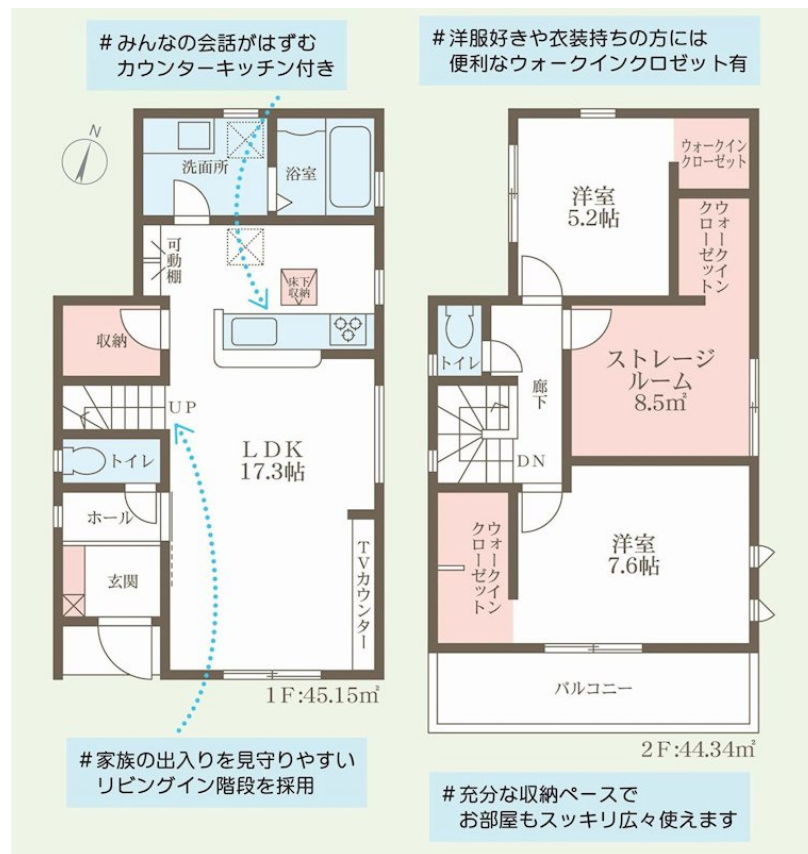
【間取り図】
