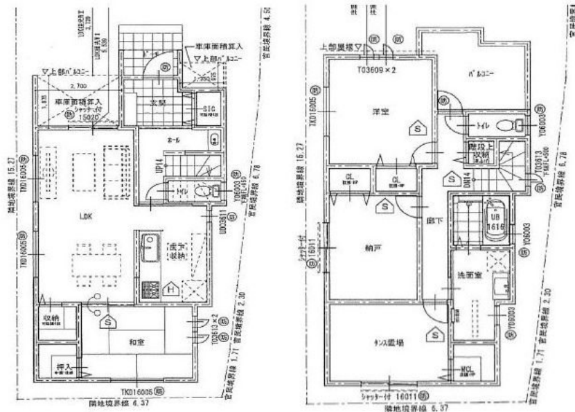
【間取り図】
