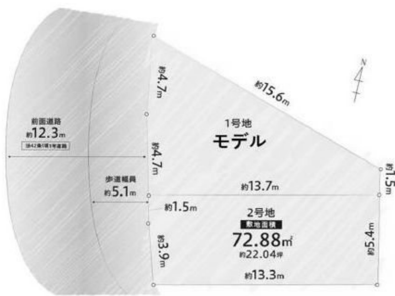
【区画図】
