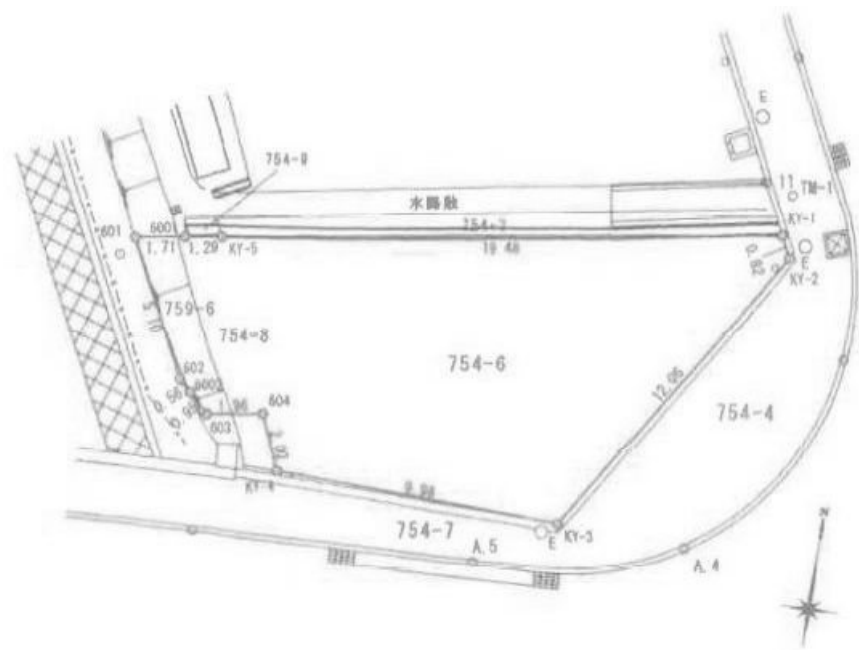
【区画図】
