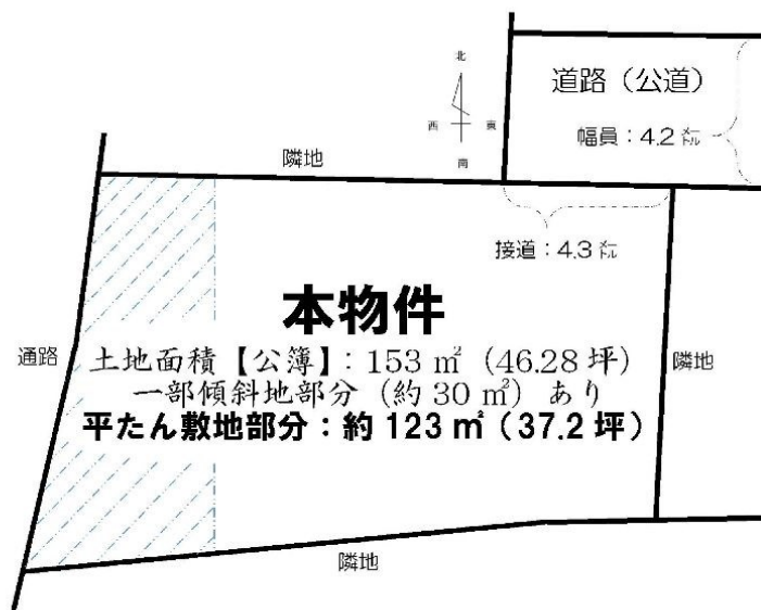
【区画図】
