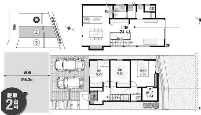
【間取り図】
