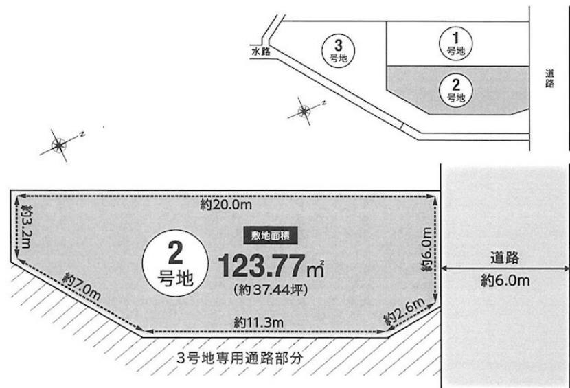
【区画図】
